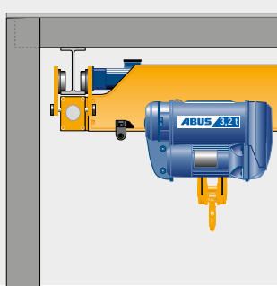
Opgebokte uitvoering Variant 2 (geoptimaliseerde haakhoogte zonder kraanliggeroversteek)
