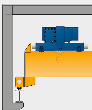
Opgebokte uitvoering Variant 4
