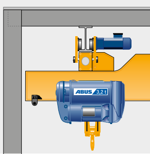
Standaard hoofdligger - aansluiting – Variant 1 B (optimalisatie haakhoogte en kataanrijmaten)
