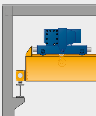
Opgebokte uitvoering Variant 3
