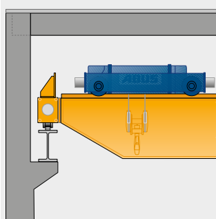
Standaard hoofdligger-aansluiting Variant 1 in combinatie met een verdiept gemonteerde loopkat
