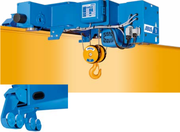
Looprollen met scharniergewricht.
