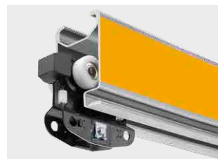
Inwendig loopprofiel met loopwerk
