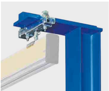
Draagarmconstructie met enkelzijdige overstek
